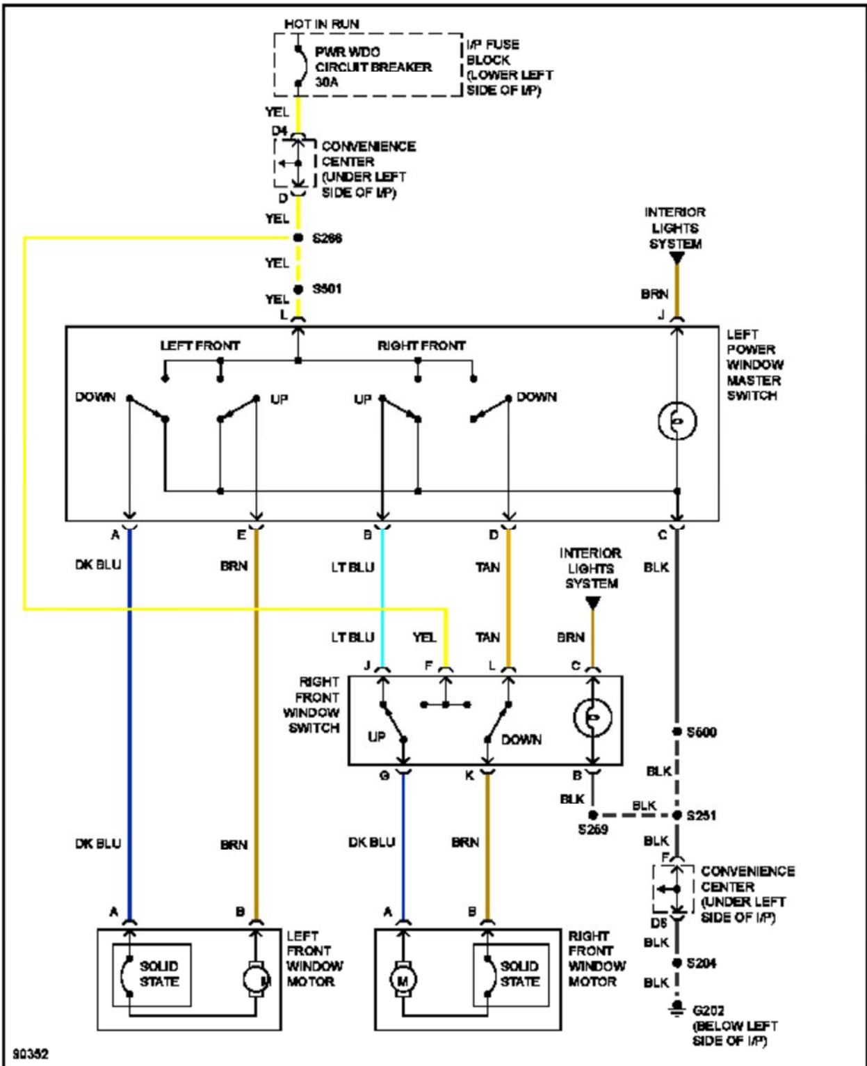
Fig. 66: Power Window Circuit, 2 Door
